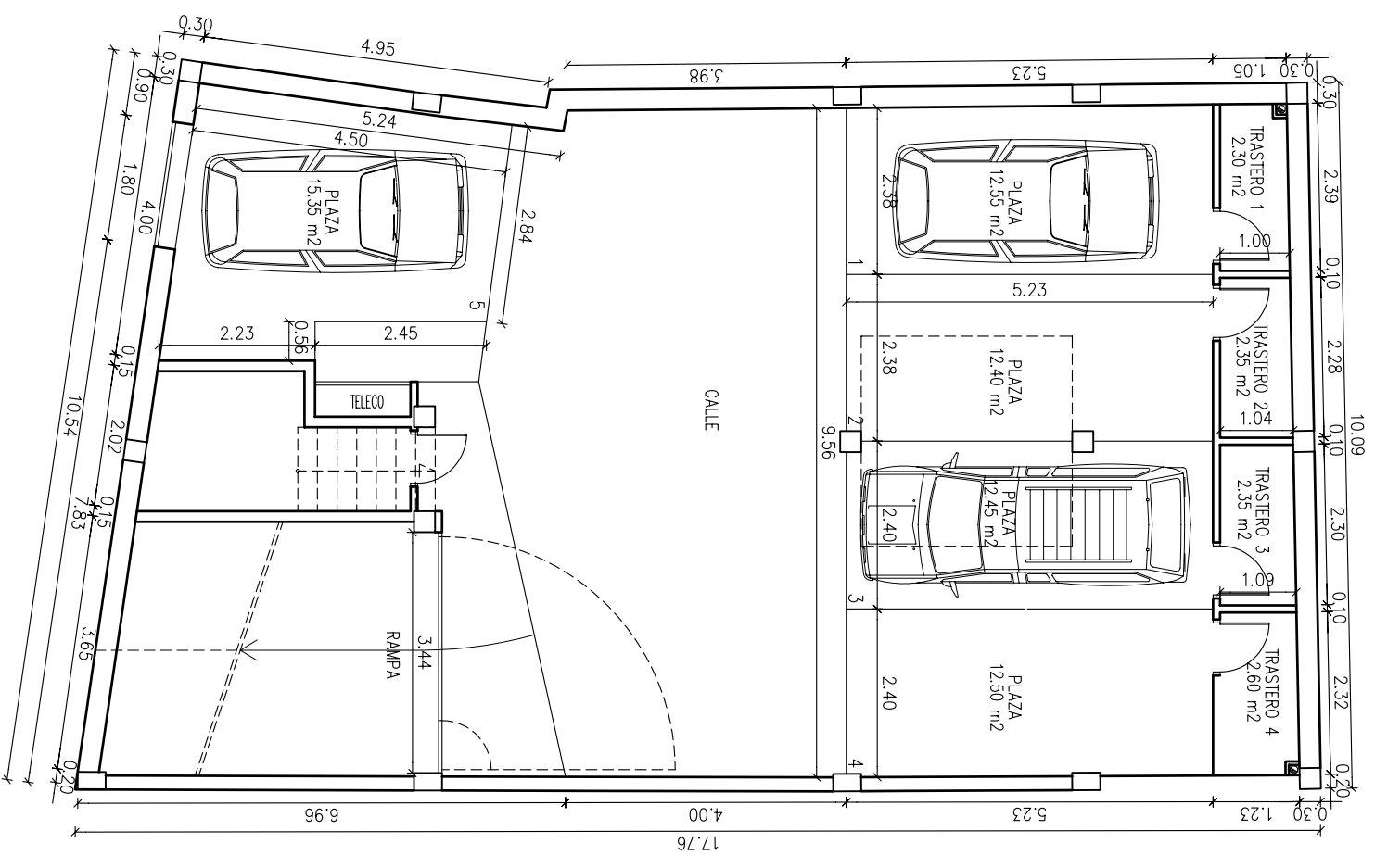
PLANTA SEMISOTANO Distribución y Superficies Escala: 1/100
